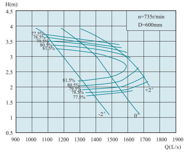
700QZ-160
