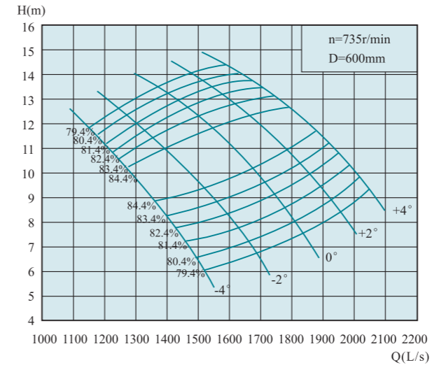
800QH-50
