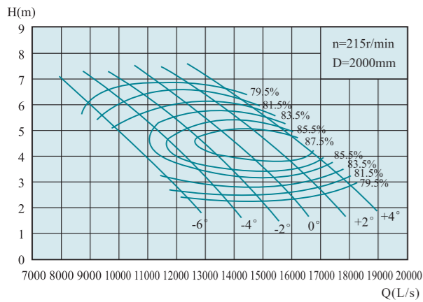
2000QZX-100
